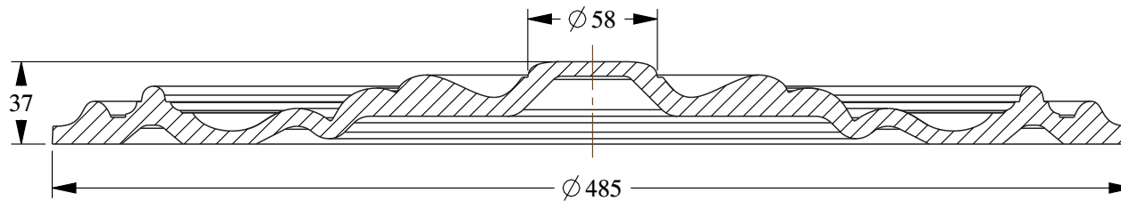
SECTION A-A
