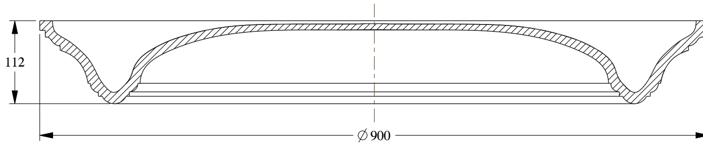
SECTION A-A
